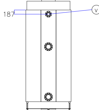
Вид сверху
