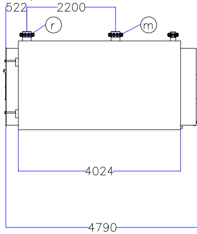
Вид справа
