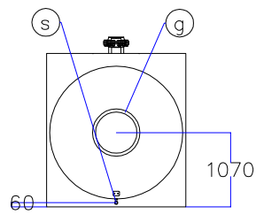
Вид сзади
