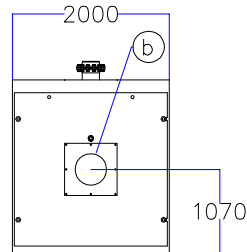
Вид спереди
